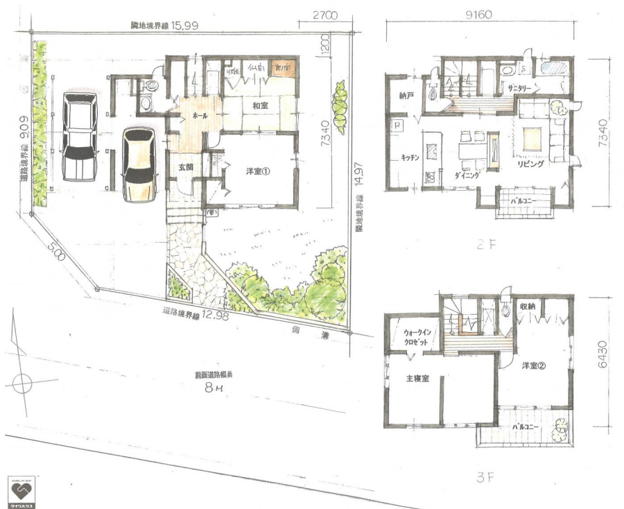
間取り
